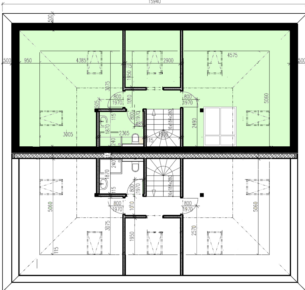
půdorys podkroví - 59,1 m 2 (76,1 m 2 )
